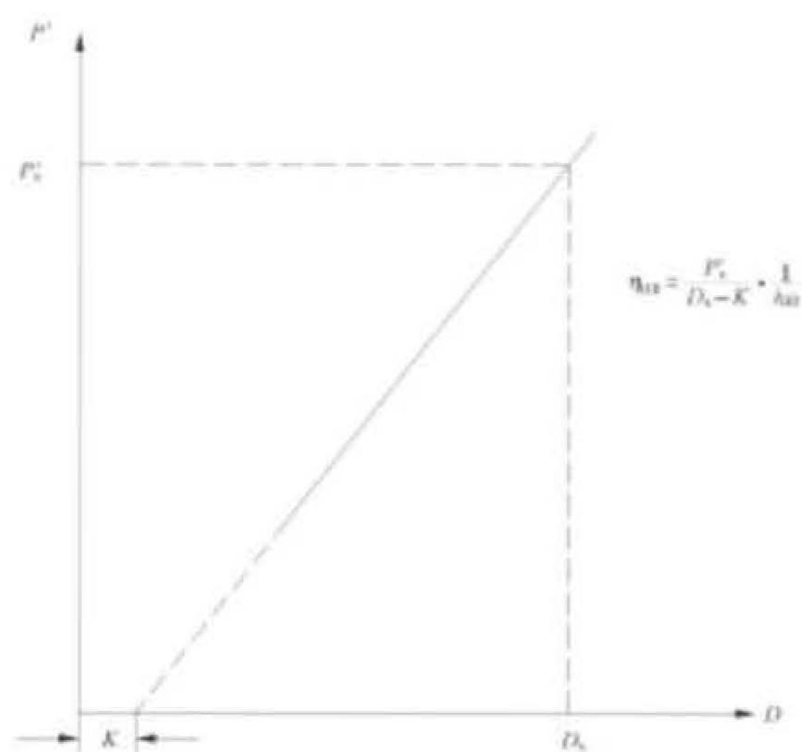
图 L.2 机械传输装置的 P' - D 关系曲线
