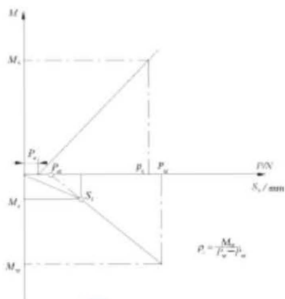
图 L.6 机械制动器 M-P/M-S r 关系曲线
