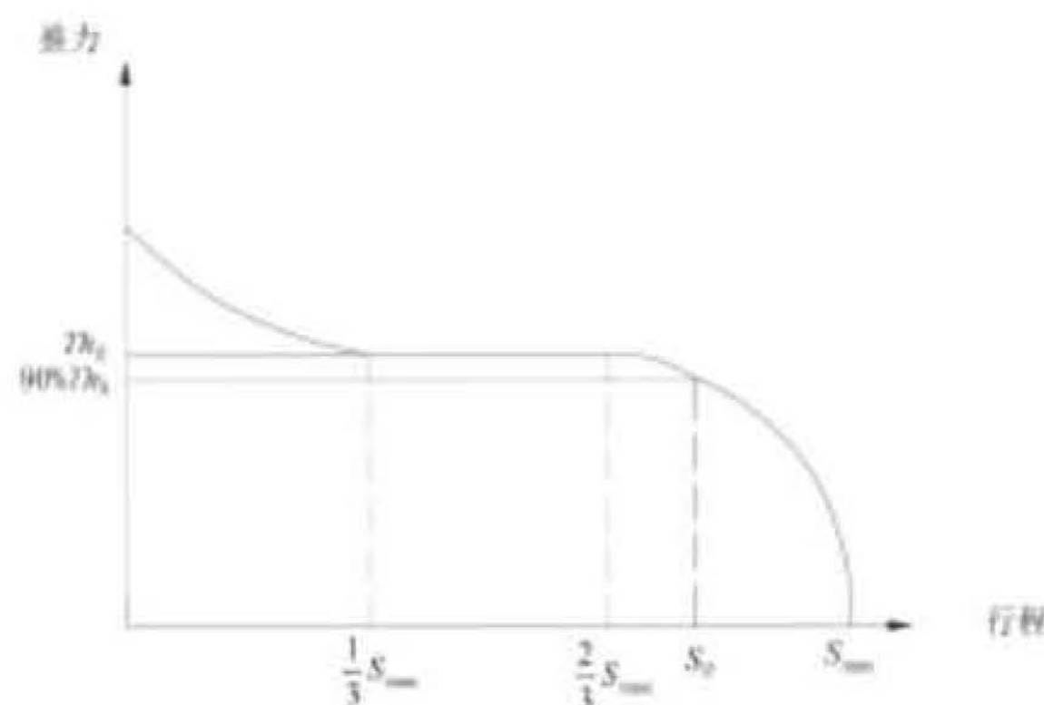
图 K.1 推力与行程的关系
