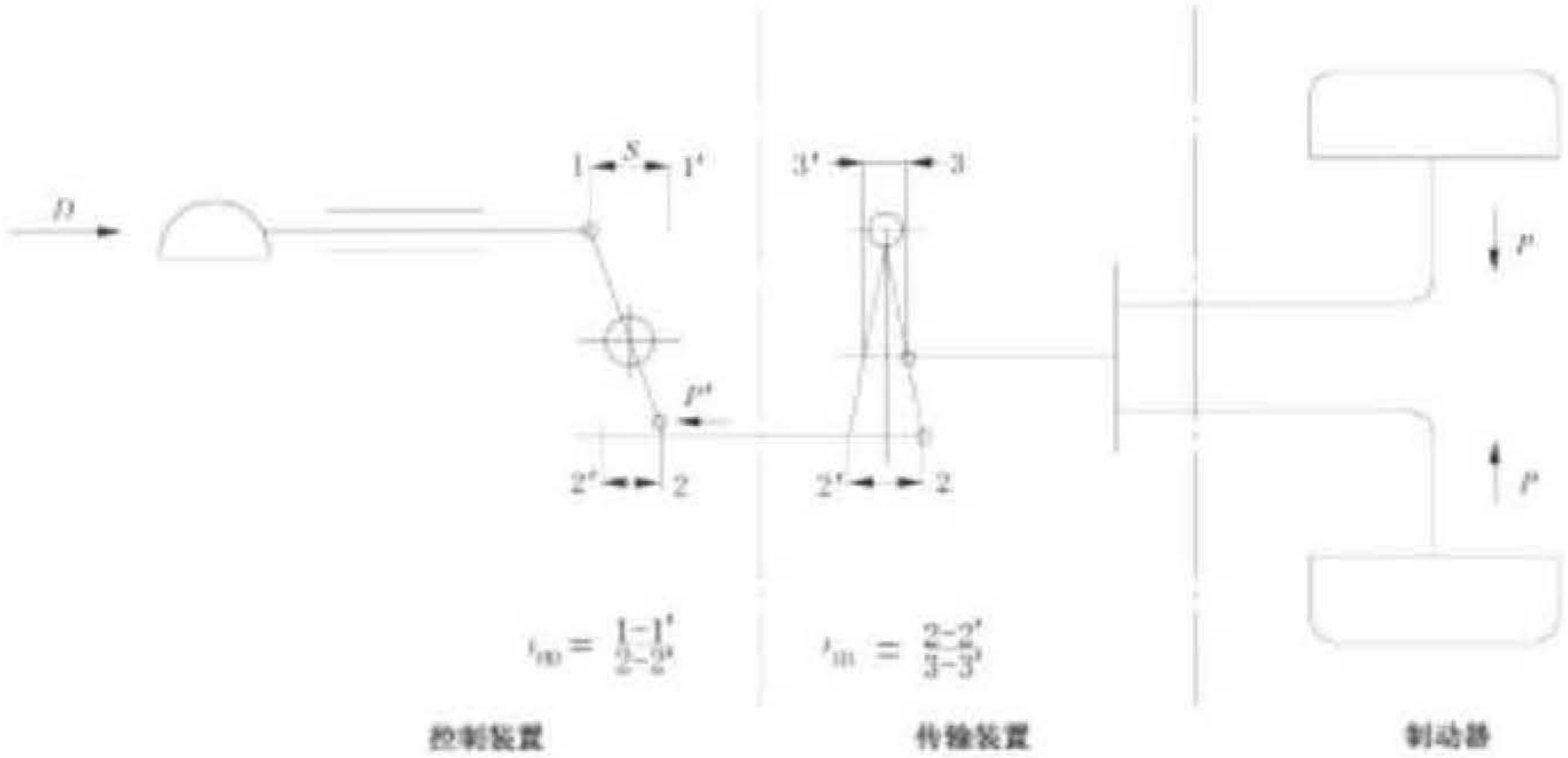
图 L.5 机械传输式制动系统组成示意图
