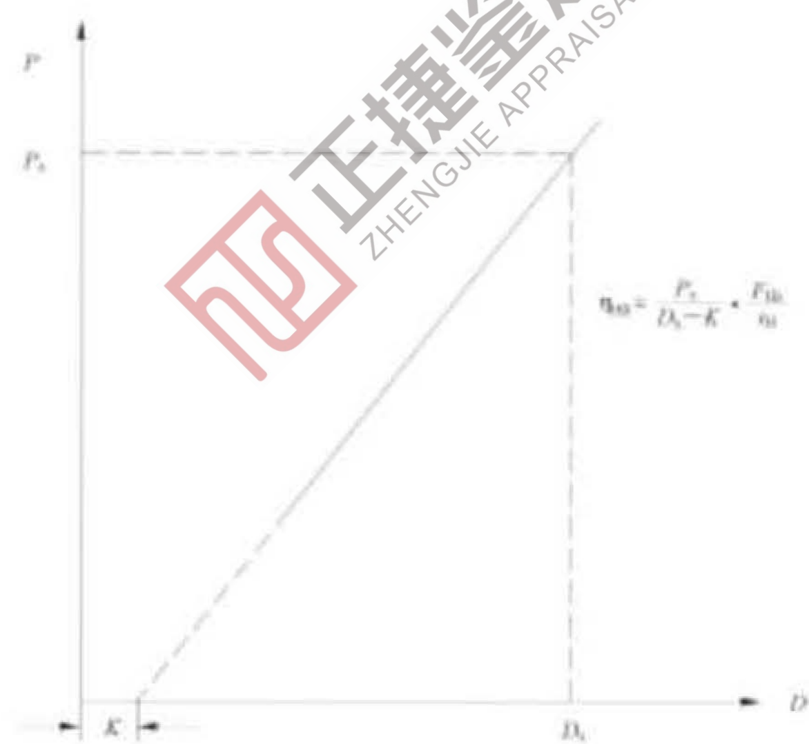
图 L.3 液压传输装置的 P - D 关系曲线
