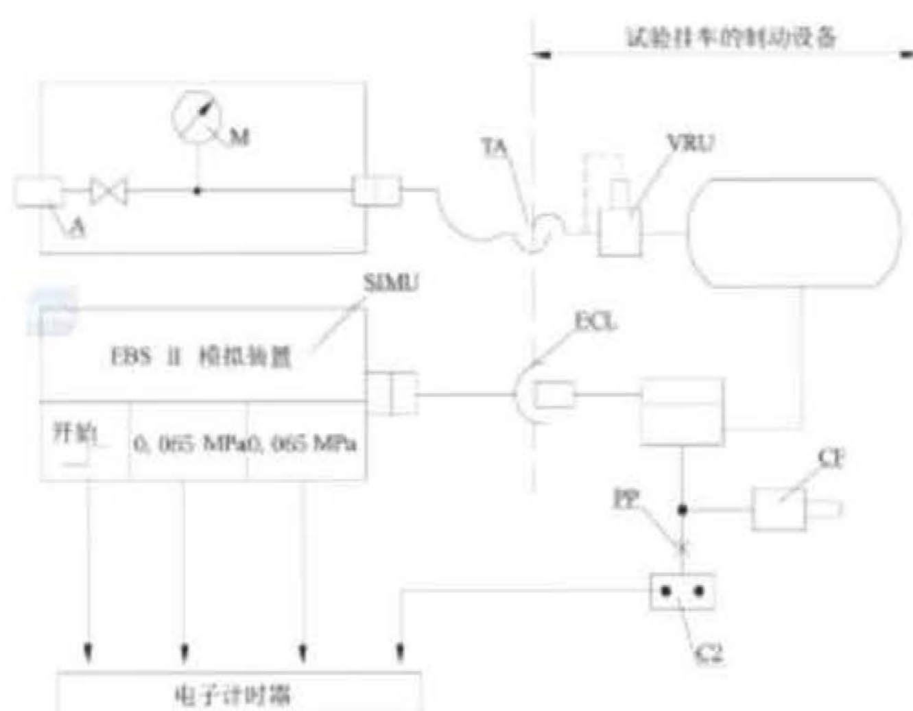
c) 电控线路模拟装置实例
